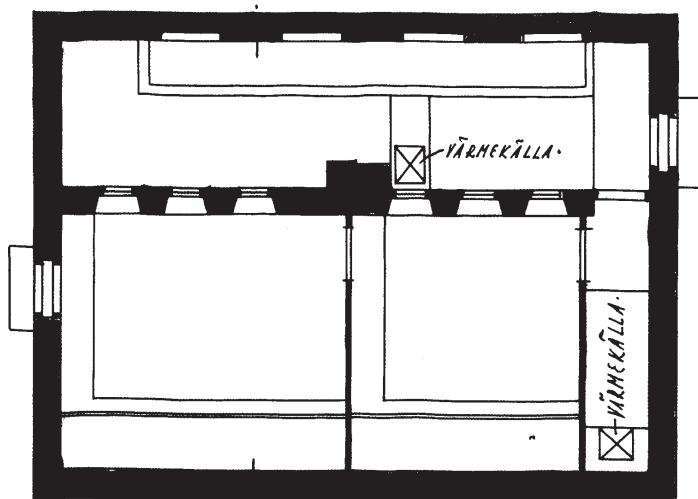
· SÖDRA · LÅNGSIDAN ·
